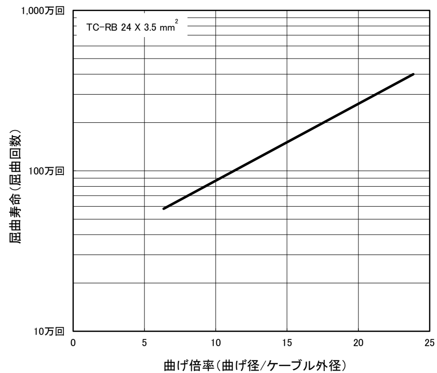
図5 丸型バンドタイプ (TC-RB) の寿命 (曲げ倍率-屈曲寿命)
