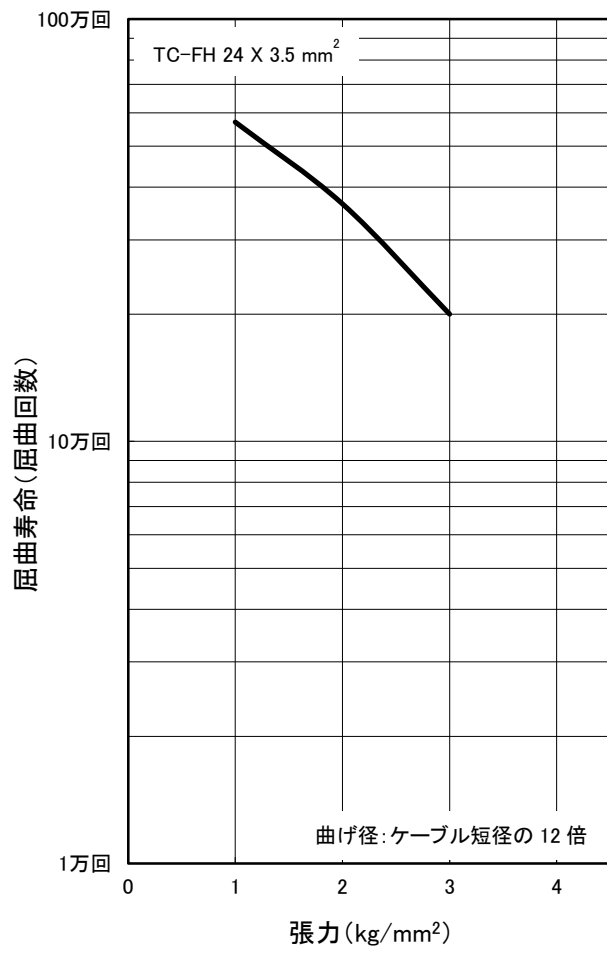
図 1 平型ハイテンションタイプ (TC-FH) の寿命 (張力ー屈曲寿命)
