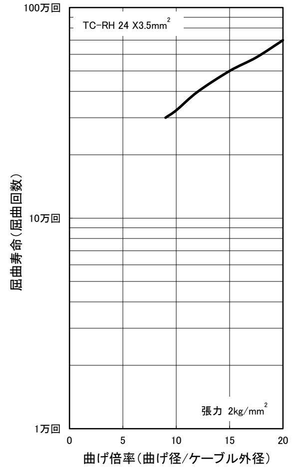
図4 丸型ハイテンションタイプ (TC-RH) の寿命 (曲げ倍率-屈曲寿命)
