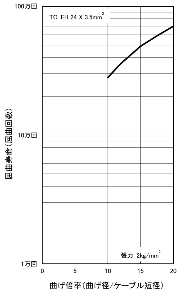
図 2 平型ハイテンションタイプ (TC-FH) の寿命 (曲げ倍率ー屈曲寿命)
