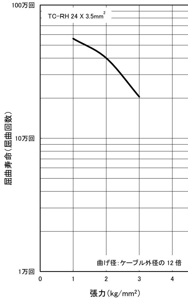
図3 丸型ハイテンションタイプ (TC-RH) の寿命 (張力-屈曲寿命)
